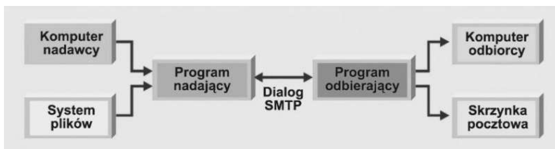
Rys.1. Schemat funkcjonowanie SMTP (Itpedia.pl, SMTP).
